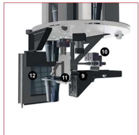
Abbildung 3 Detailansicht des Ausgabegeräts in Position
